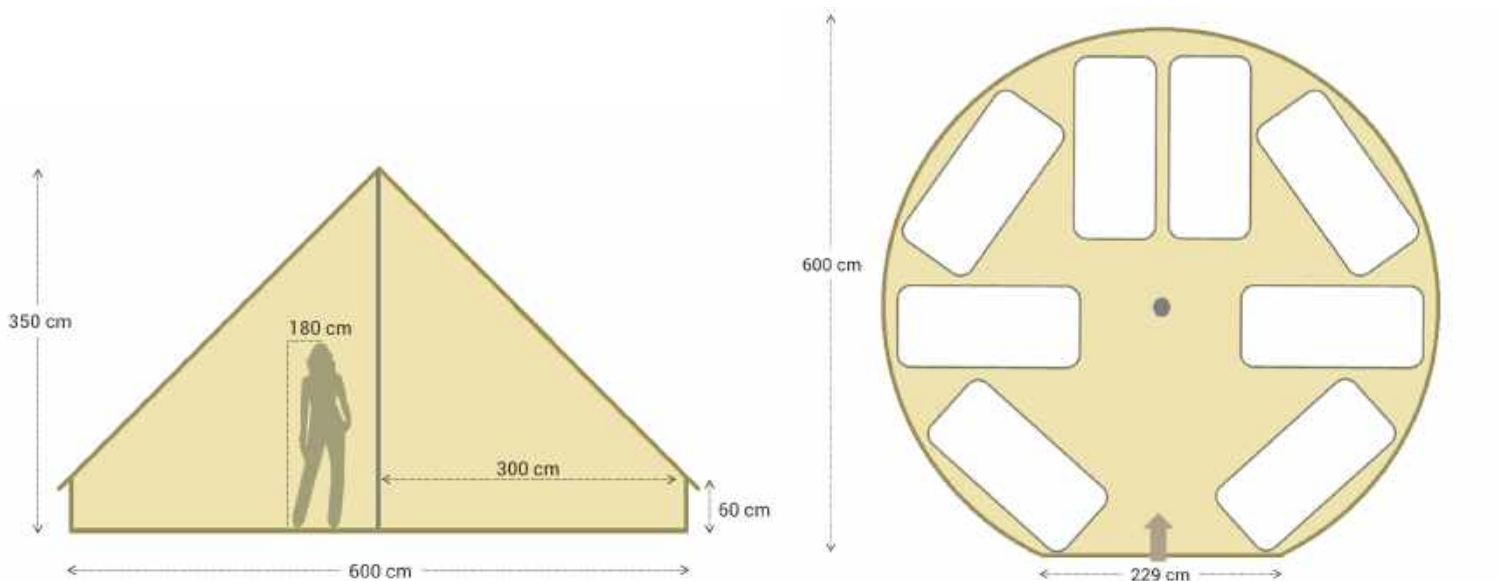
Coupe latérale
